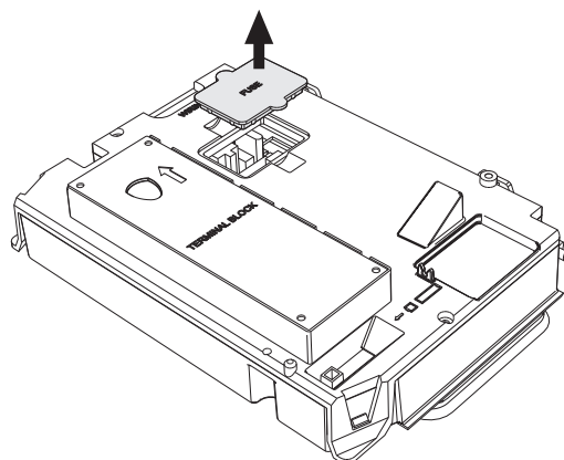
fig. 53 - Alloggiamento fusibile
