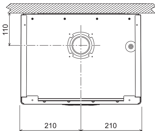
fig. 56 - Vista dall'alto
