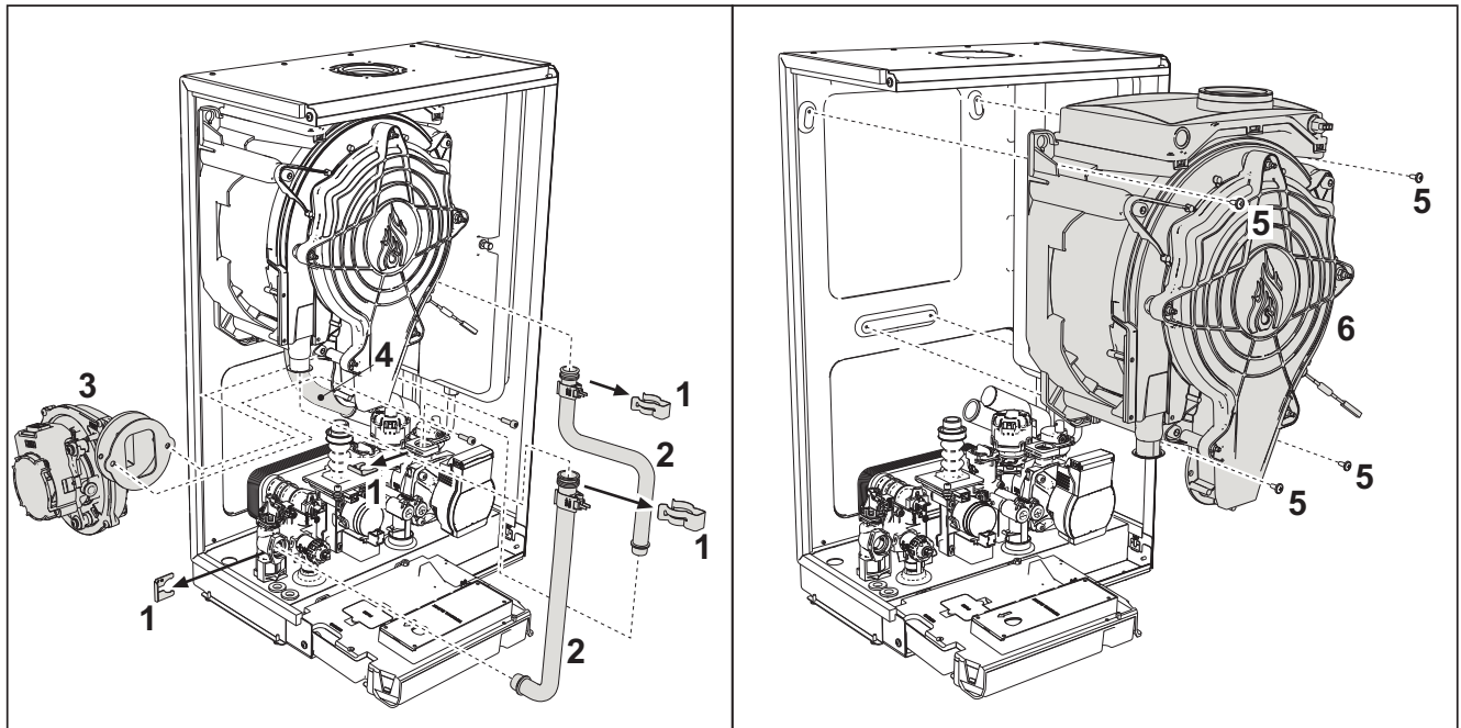
fig. 41 - Scambiatore principale
