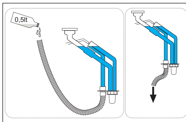
fig. 29 - Collegamento scarico condensa
