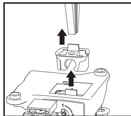
рис. 36- Замена газовой диафрагмы
