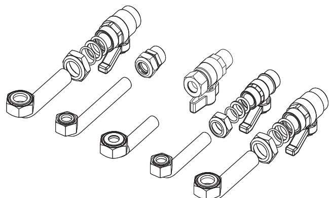
рис. 18- Гидравлический комплект
