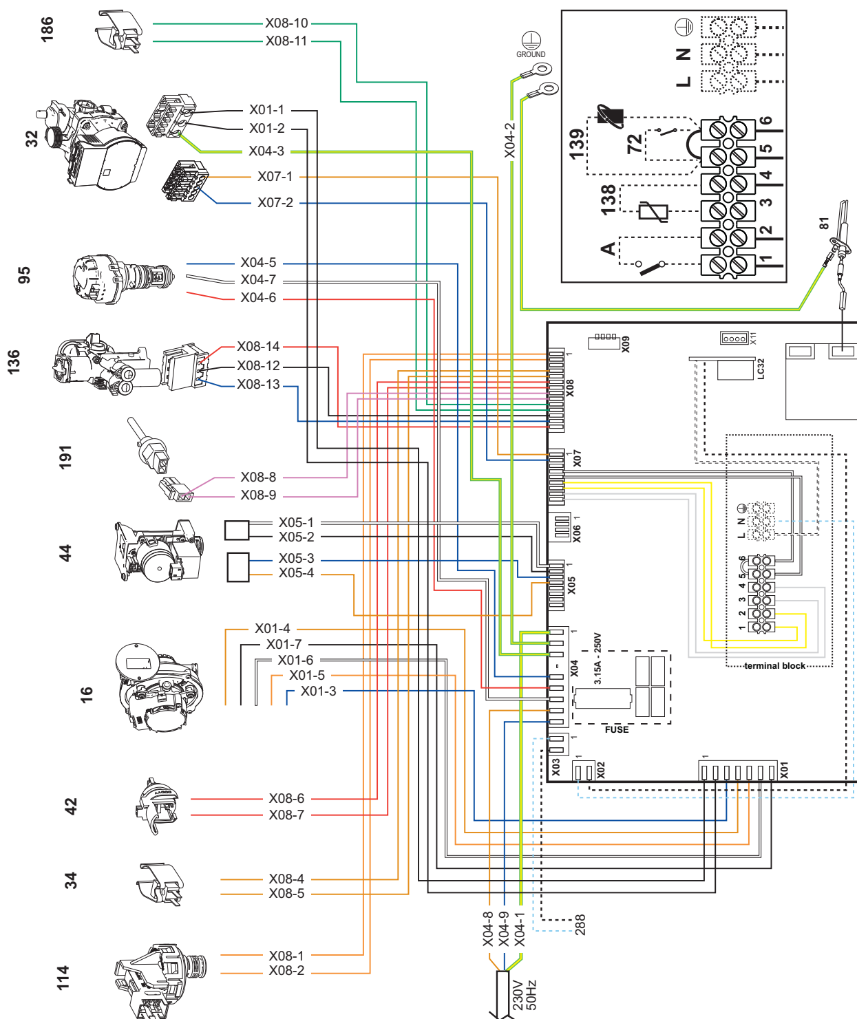
fig. 63 - Schema elettrico
