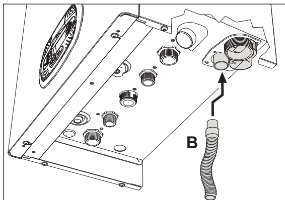
рис. 29- Подсоединение трубы для слива конденсата
