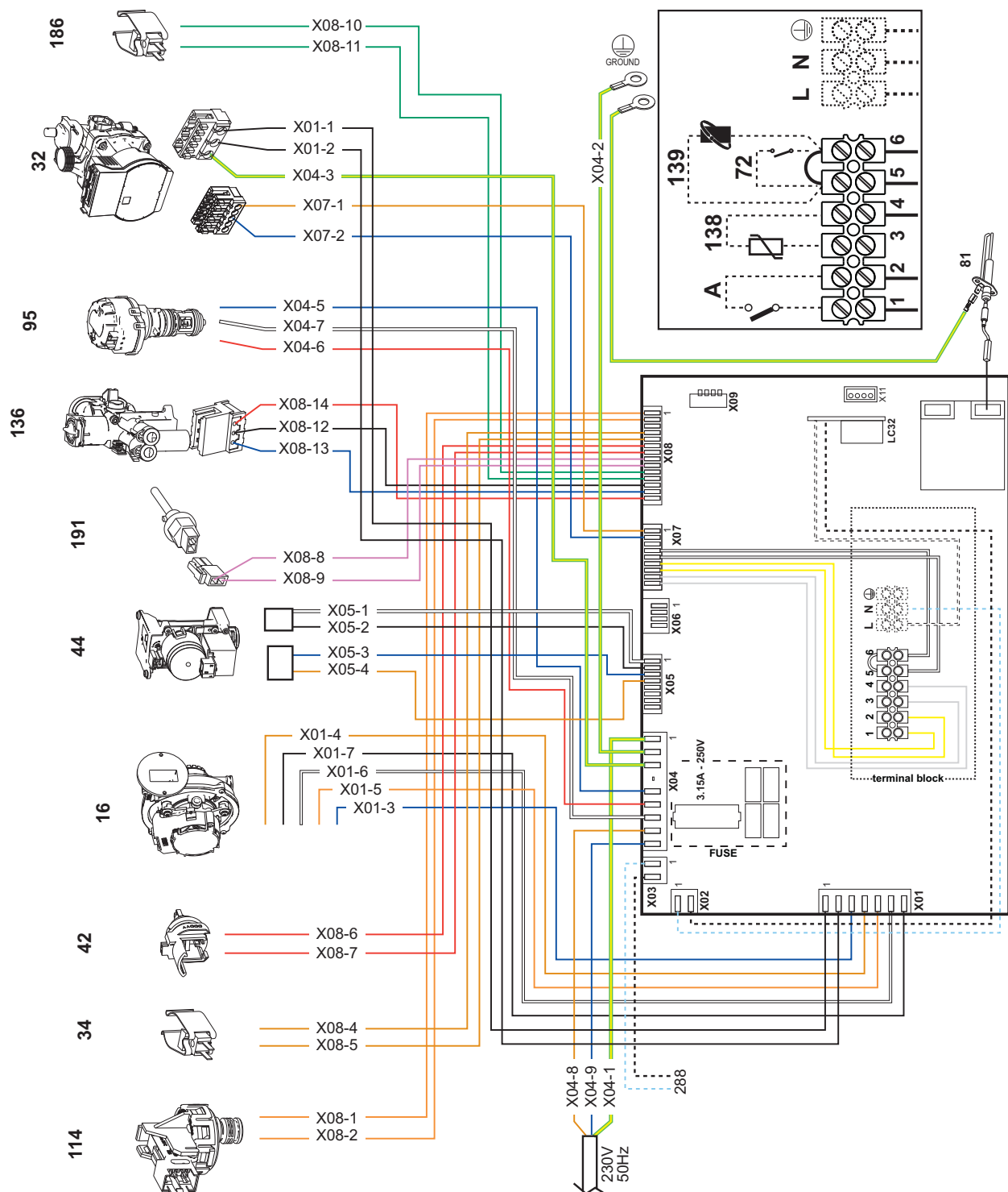
рис. 63- Электрическая схема
