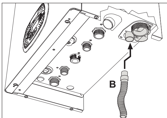
fig. 29 - Collegamento scarico condensa
