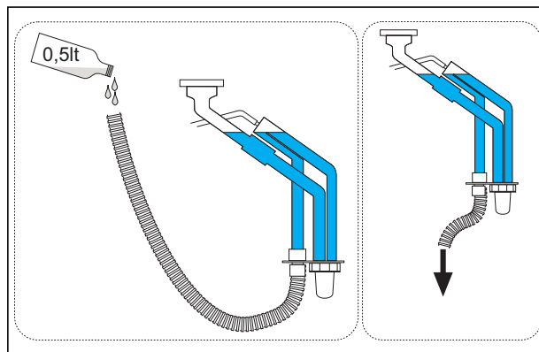
рис. 29- Подсоединение трубы для слива конденсата
