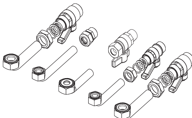
fig. 18 - Kit idraulico
